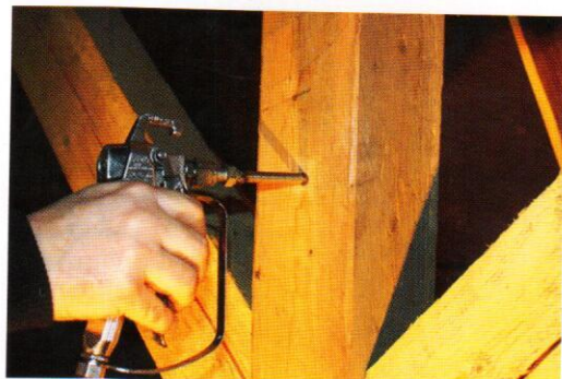
Tlaková injektáž
